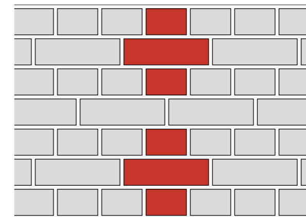
KREUZVERBAND
