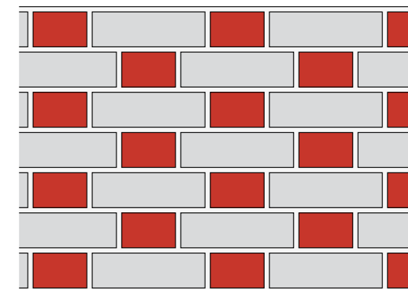
FLÄMISCHER VERBAND
