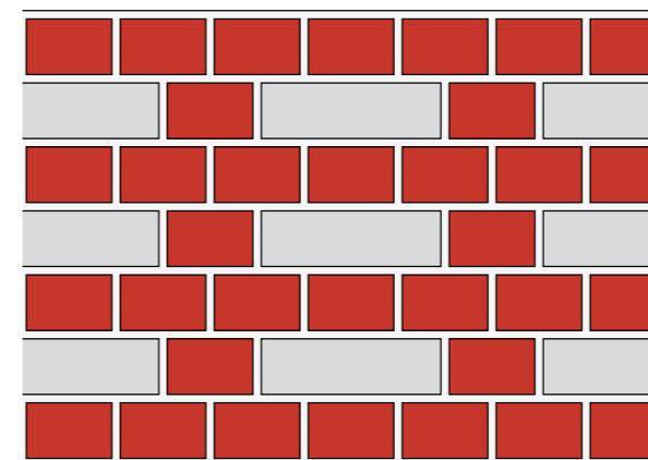
HOLLÄNDISCHER VERBAND
